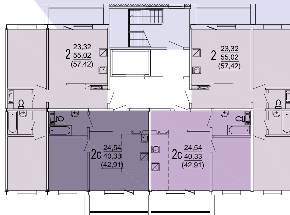
типовой этаж
